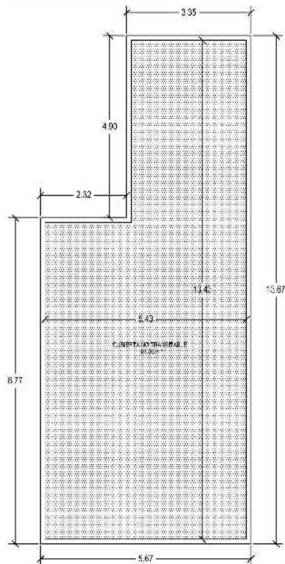
PLANTA CUBIERTA
