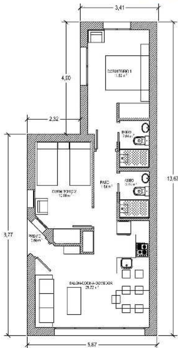
PLANTA BAJA
